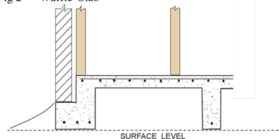
Fig 2 Waffle Slab
